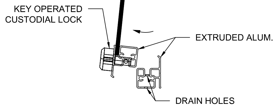
1 D1 HEADER AND SILL SECTION SCALE: 1"=0'-2"
